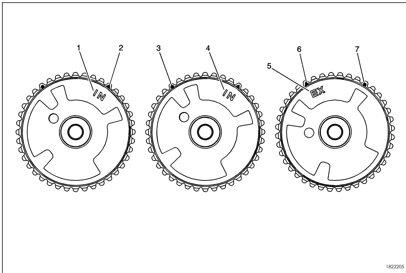
凸轮轴位置执行器正时标记
